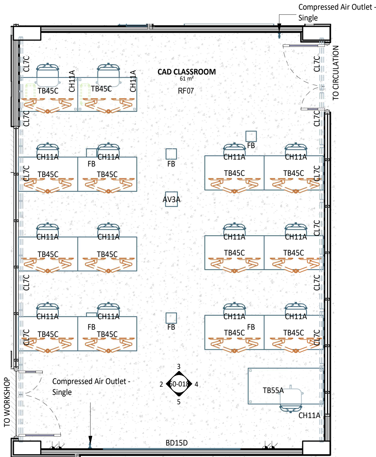
1 PLAN DETAIL 30-01 1 : 50
